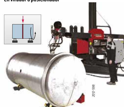
Soldadura circular con columna y brazo en virador o posicionador
