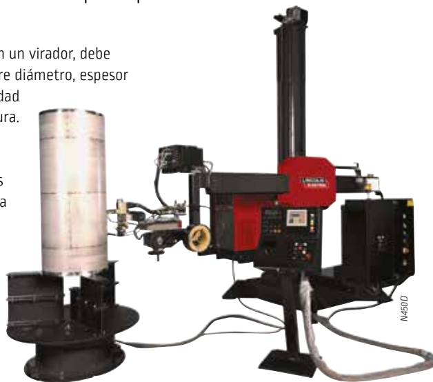
Mesa giratoria estandar de 5 a 30 T Hasta 4500 mm diámetro
